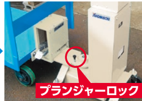
連結完了後、プランジャーロックを解除して操作してください
