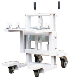
123 ハンドリフト(手巻) ●荷重200kg ●巻き揚げタイプ ●テーブル式
